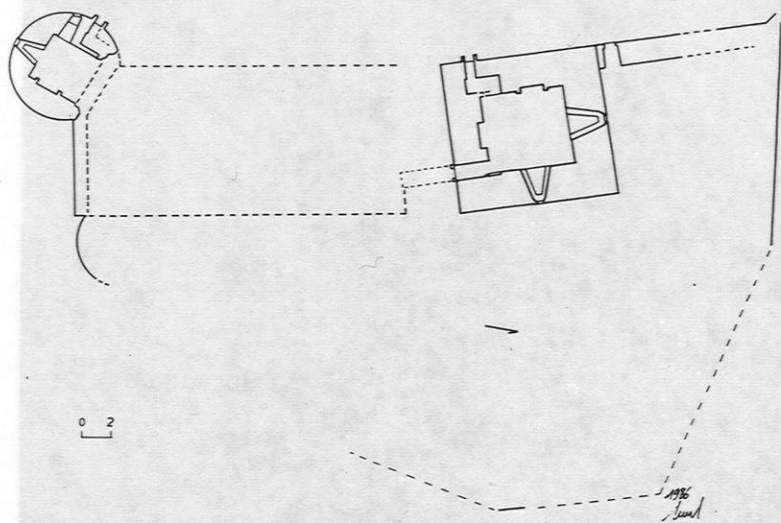
Cuguen (Ille-et-Vilaine). La Roche-Montbourcher. Plan des vestiges au niveau du premier étage.
