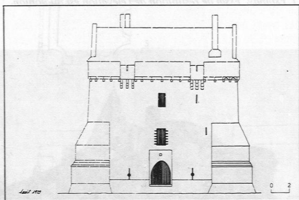
Créhen (Côtes-d'Armor) La Touche-à-la-Vache. Essai de restitution de l'élévation ouest.
