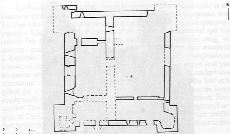
Créhen (Côtes-d'Armor) La Touche-à-la-Vache. Plan du rez-de-chaussée.
