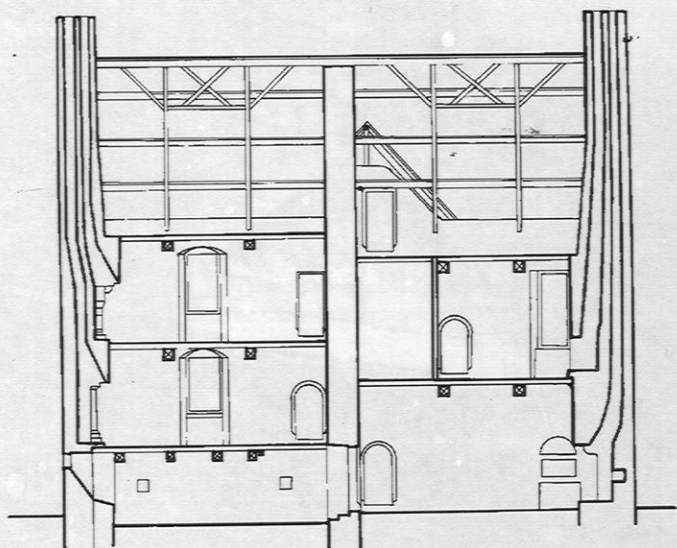
Coupe longitudinale du corps de logis
