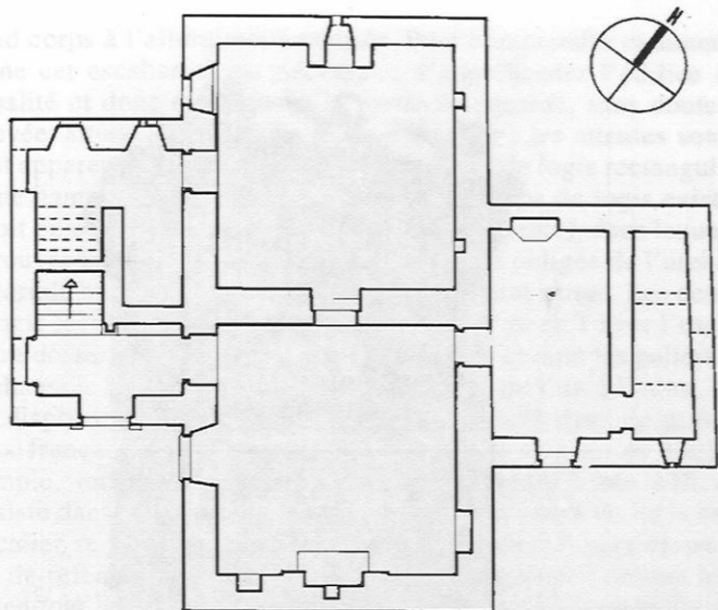
Plan au rez-de-chaussée
